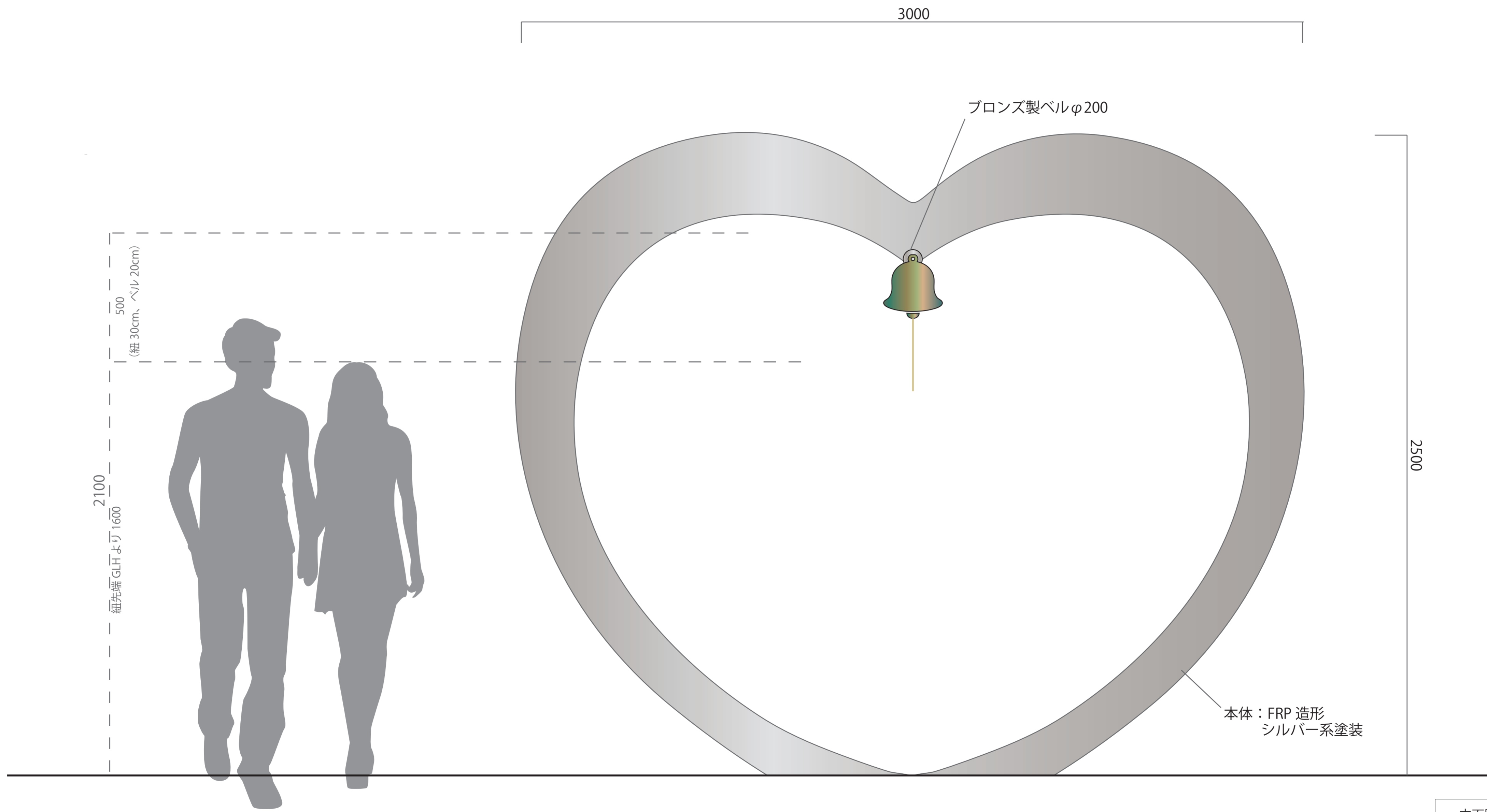
立面図
